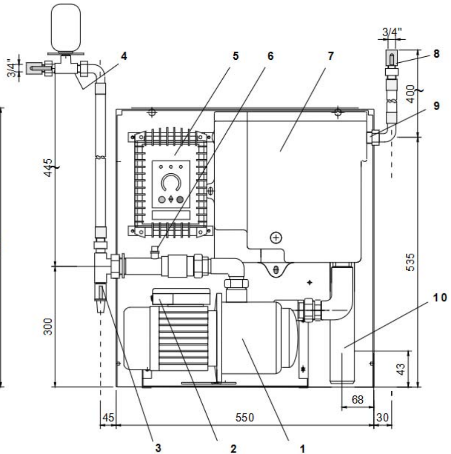
Frontansicht
