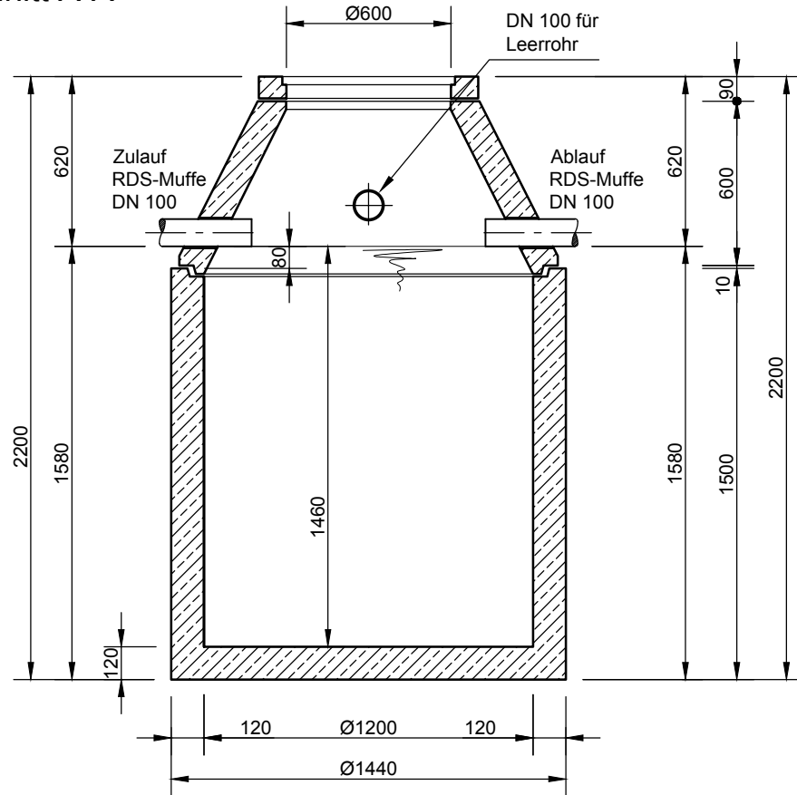
Grundriss
