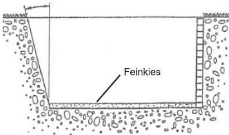
1a Böschungswinkel nach UVV einhalten oder Verbau einbringen
